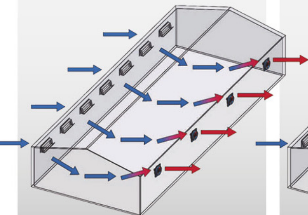
Ventilazione TRASVERSALE
